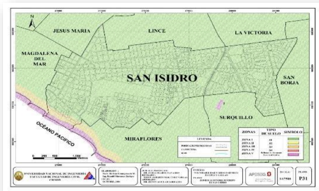
Figura 9. Zonificación Geotécnica Sísmica
