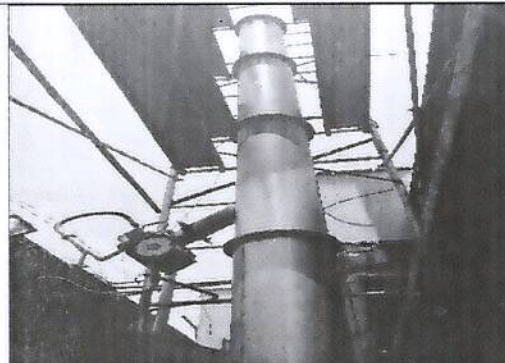
Sistema de depuración (Chimenea ecológica)
